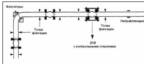
Рис. 9. Пример установки гибкой вставки типа ZKB.
