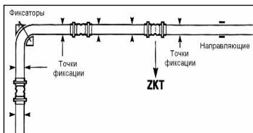
Рис. 8. Пример установки гибкой вставки типа ZKT.
