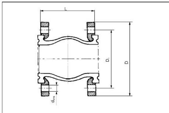
Рис. 11. Габаритные размеры гибкой вставки типа ZKB.
