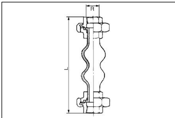
Рис. 10. Габаритные размеры гибкой вставки типа ZKT.
